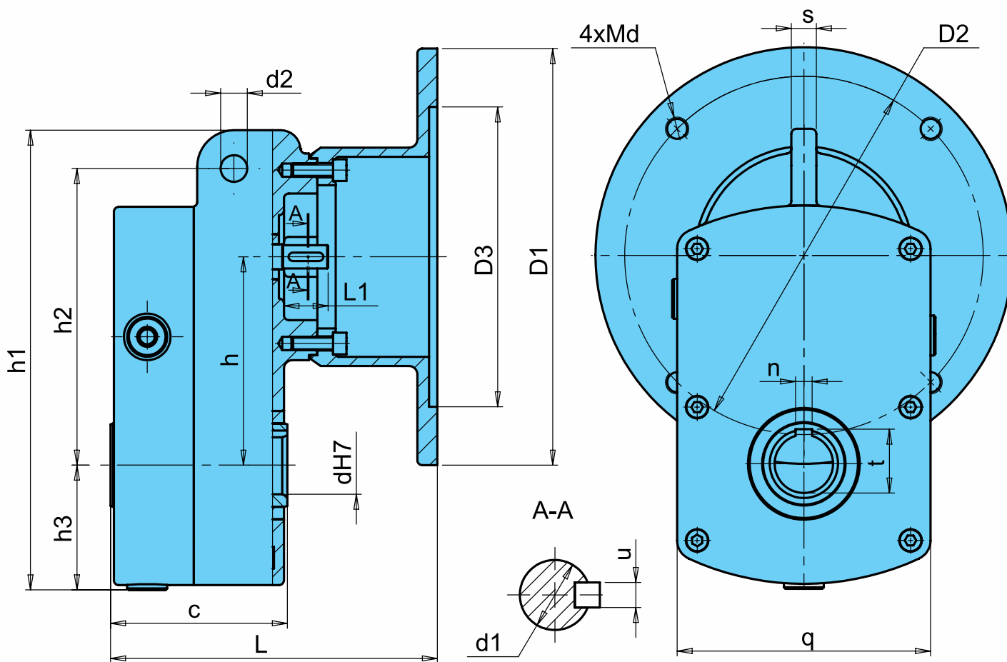
Габаритно-присъединителни размери / Габаритно-присоединительные размеры
