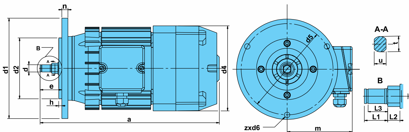
Габаритно-присъединителни размери / Габаритно-присоединительные размеры
