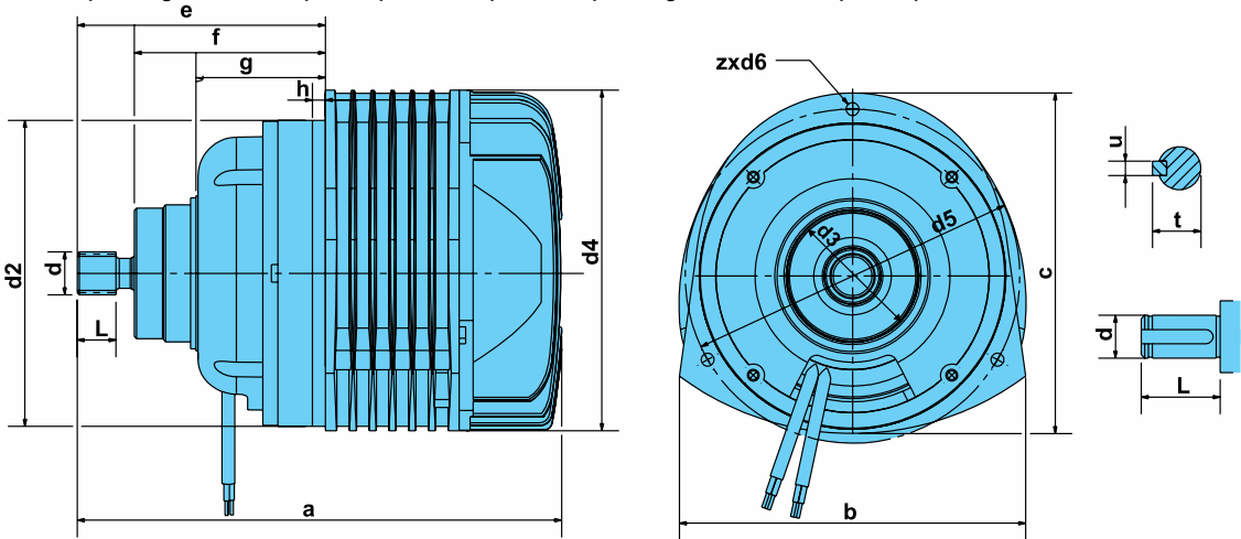
Габаритно-присъединителни размери / Габаритно-присоединительные размеры
